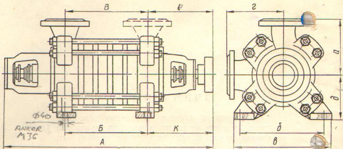
Рис. 1. Габаритные размеры насосов ЦНС 180-85...425, ЦНСМ 180-85...425; ЦНС 300-120...600, ЦНСМ 300-120...600
