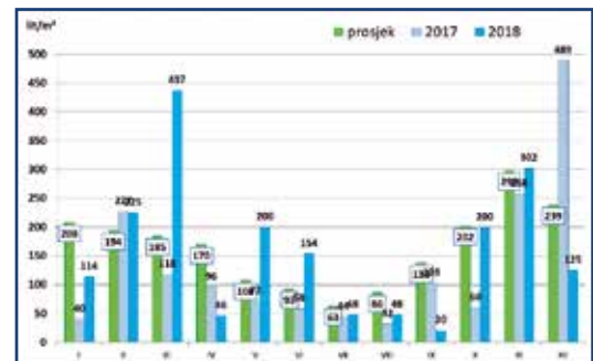
Dijagram 1: Količine padavina slivno područje rijeke Zete
