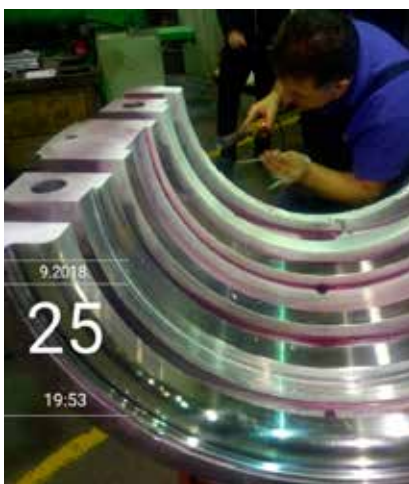
Prijemna ispitivanja generatorskog ležaja
